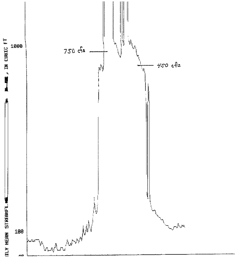
USGS 13127000 BIG LOST RIVER BL MACKAY RES NR MACKAY ID
