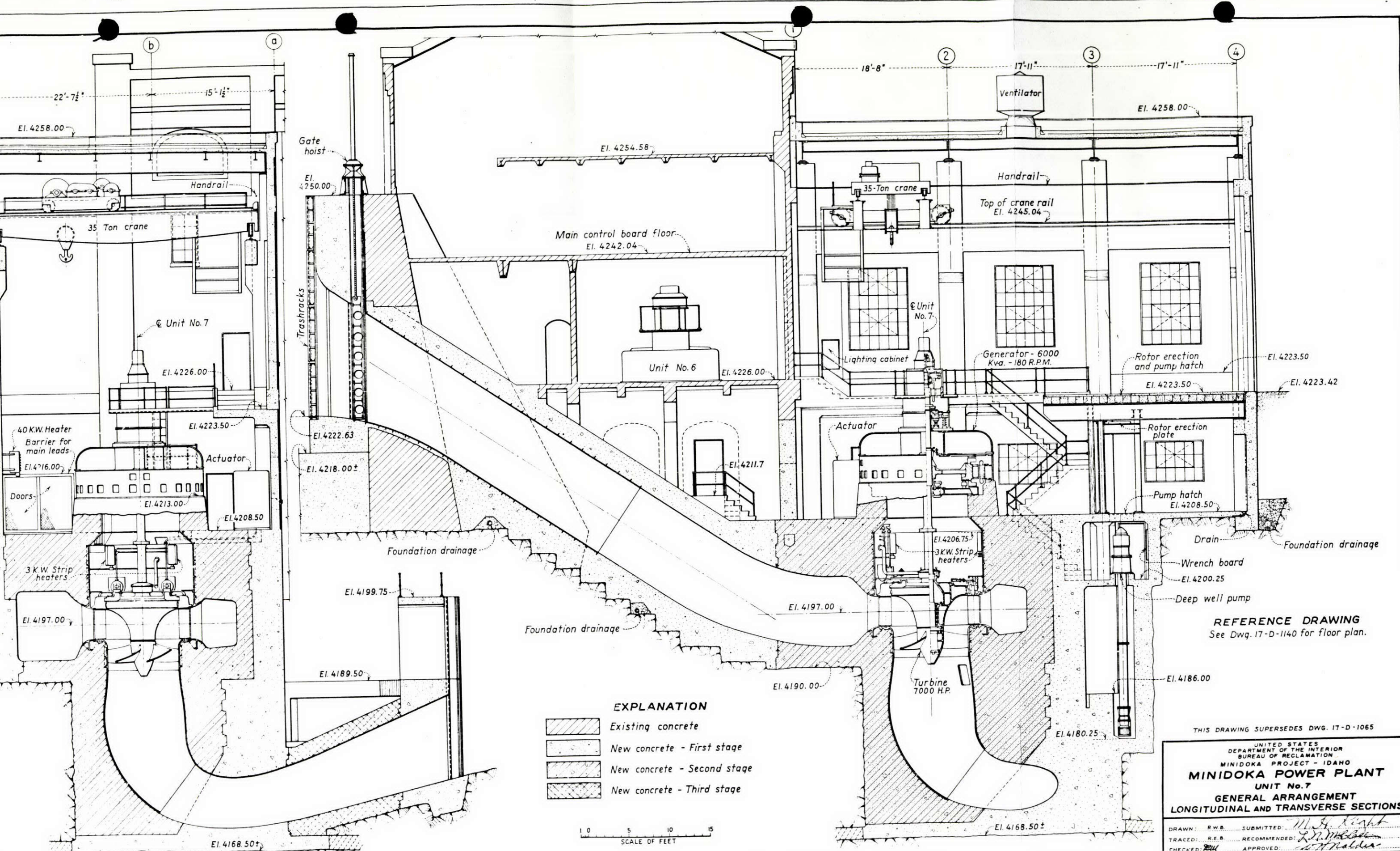
LONGITUDINAL SECTION B-B (1140)
