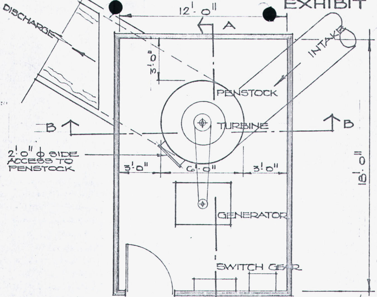
• FLOOR PLAN •
