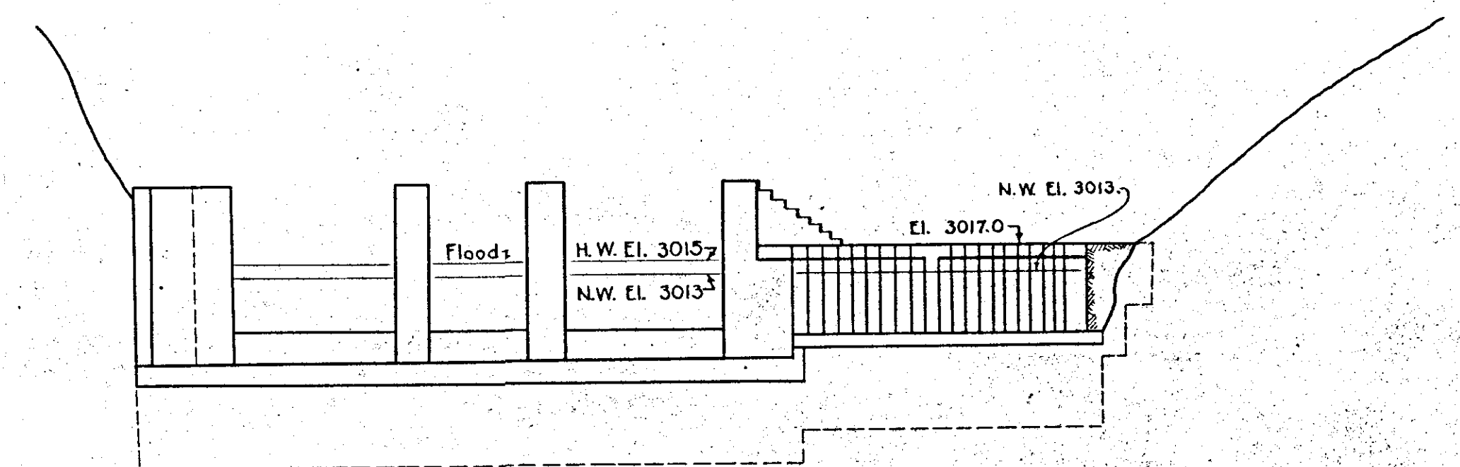
SECTION B-B Scale: 1" = 20'
