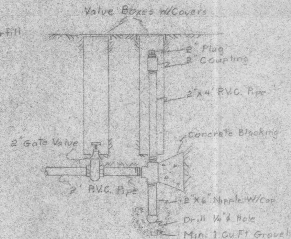
BLOWOFF ASSEMBLY N.T.S.
