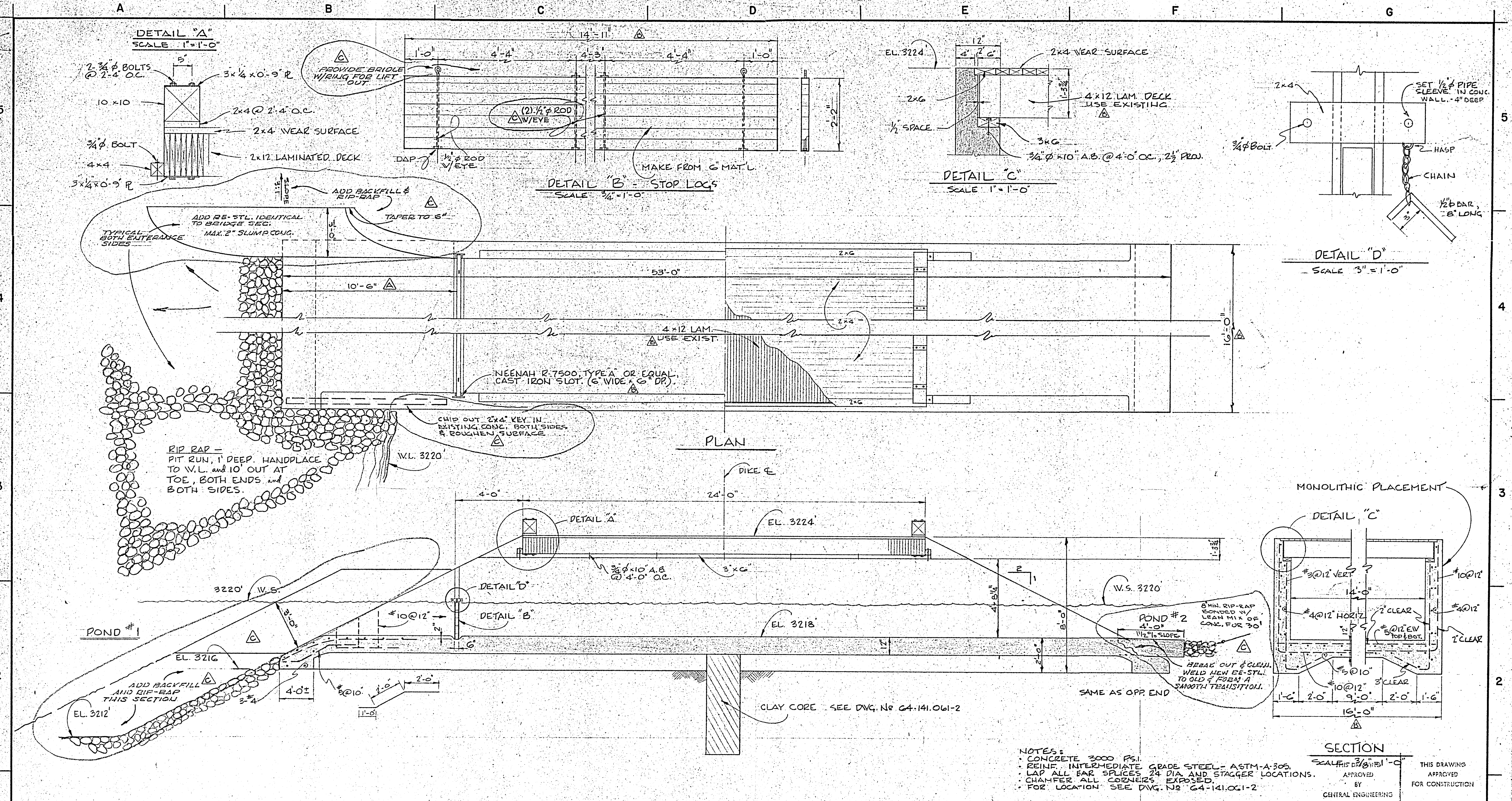
LONGITUDINAL SECTION SCALE 3/8" = 1'-0"
