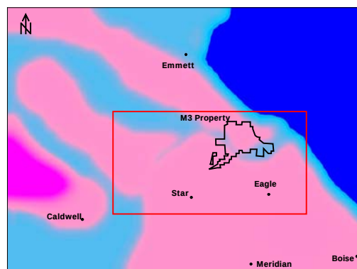
(B) Model 2 Layer 4 K (ft/d)
