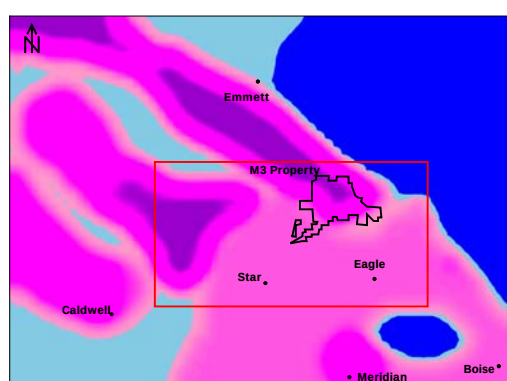
(D) Model 4 Layers 6-7 K (ft/d)
