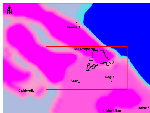
(B) Model 3 Layer 4 K (ft/d)
