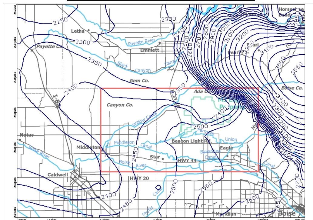
(D) Quasi-Steady-State-Model 4 potentiometric surface for layer 5
