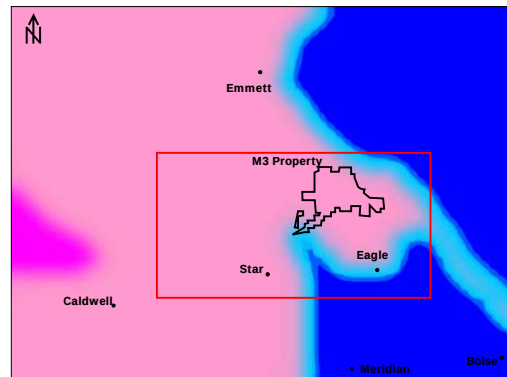
(B) Model 4 Layer 4 K (ft/d)
