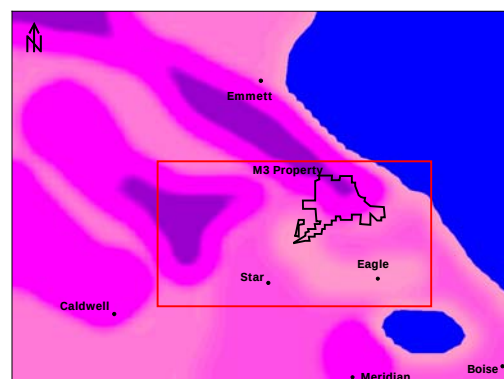
(D) Models 5a-d & 6 Layers 6-7 K (ft/d)
