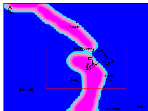
(D) Model 3 Layer 7 K (ft/d)
