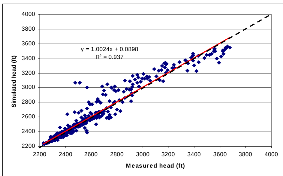
(D) Quasi-Steady-State Model 4
