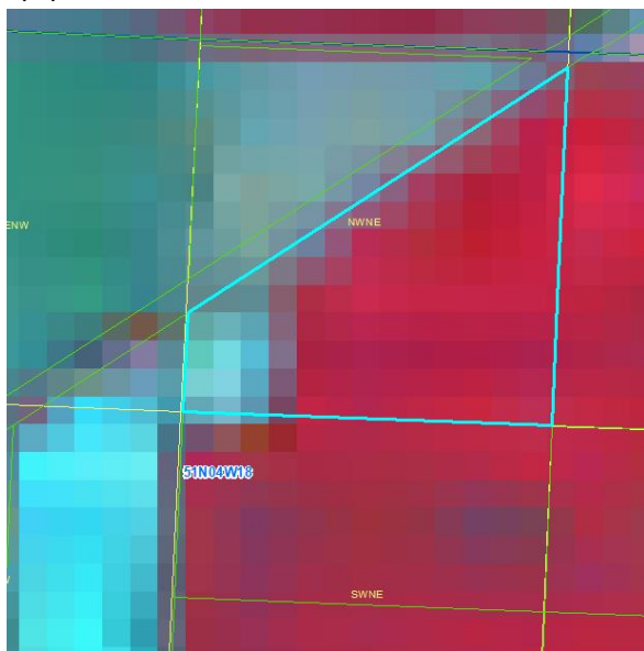
7/1/2014 LandSat
