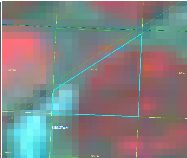
7/4/2015 LandSat
