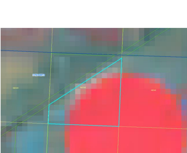
9/11/2017 LandSat
