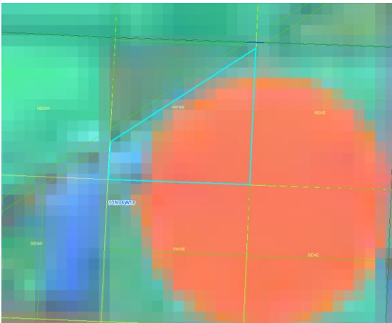
5/3/2016 LandSat
