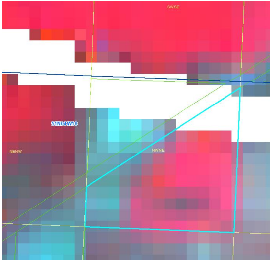
6/23/2020 LandSat
