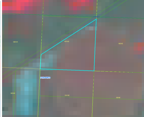
8/23/2016 LandSat
