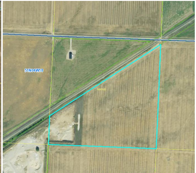
2013 NAIP
