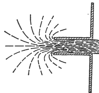
Fig. 44. Reentrant tube.
